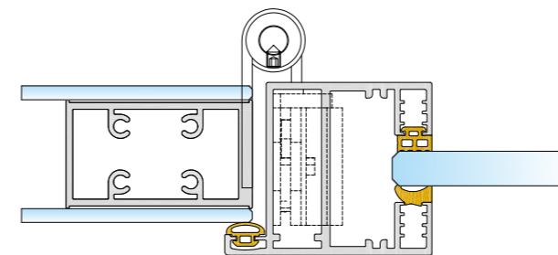
GlassDesign | Türzarge P10 | Just 3D | bis 34 dB
