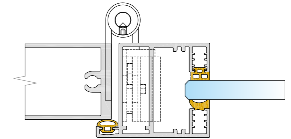
Aluminium | Türzarge P10 | Just 3D | bis 37 dB
